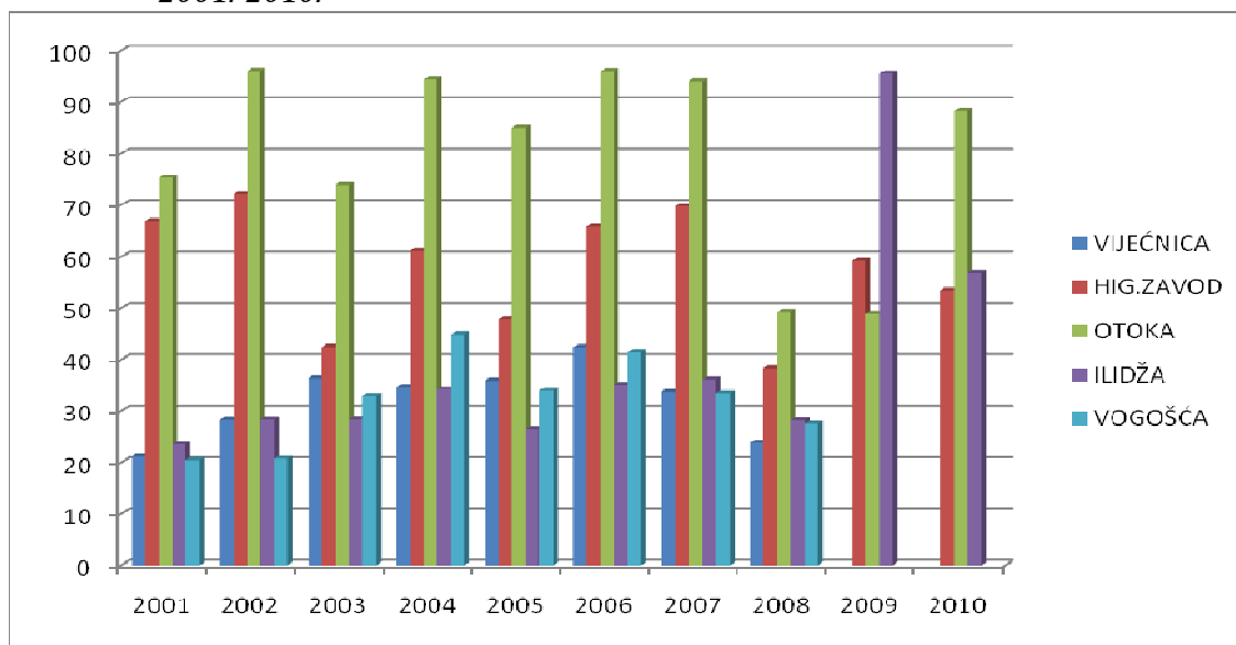
Grafikon 5. Kretanje koncentracije čađi prema godinama i različitim lokacijama, u periodu 2001.-2010.
