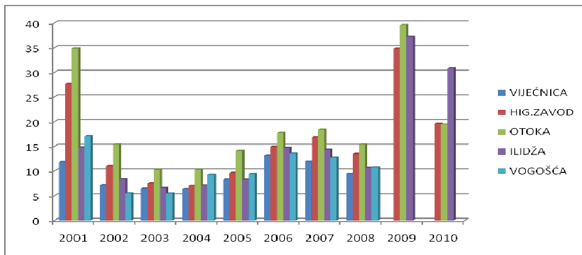
Grafikon4. Kretanje SO 2 prema godinama i različitim lokacijama, u periodu 2001.-2010.
