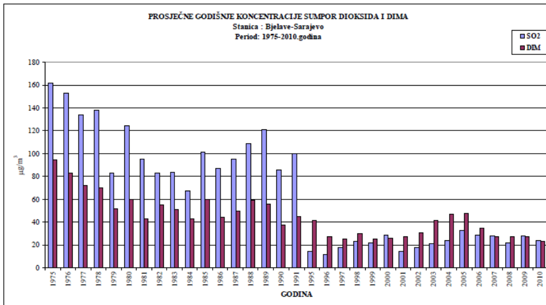
Grafikon 3. Prosječne godišnje koncentracije SO 2 i dima, mjerene na M.S. Bjelave u periodu 1975.-2010.
